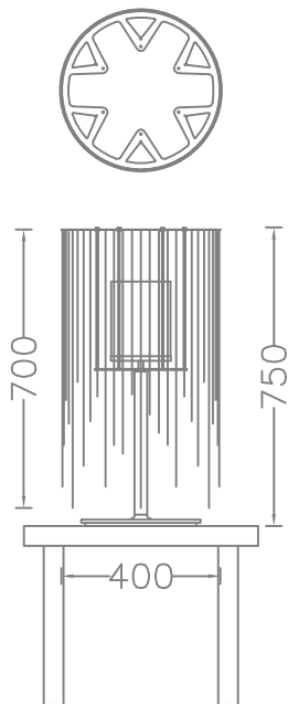
CIR-WIL-400(LRG)-TBL
